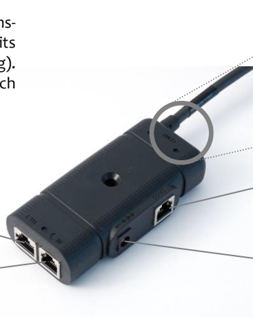
ISDN-KIT bestehend aus ISDN Modem, ISDN-Kabel und Verbindungsclip (optional erhältlich)
